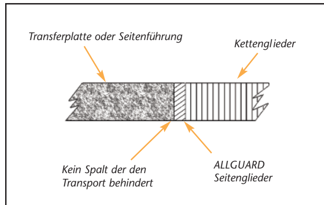
ABB. 4) ALLGUARD TRANSPORTZAHNKETTE
