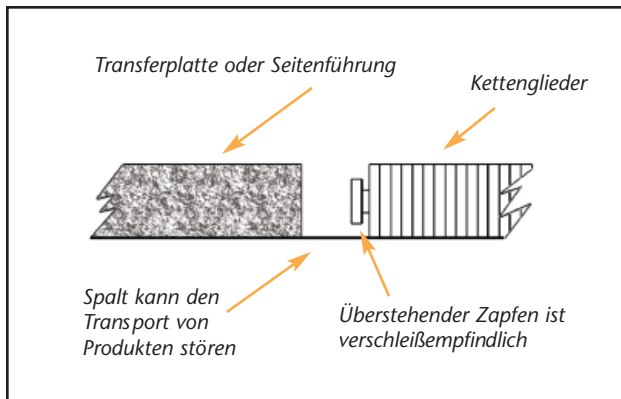
ABB. 3) HERKÖMMLICHE TRANSPORTZAHNKETTE
