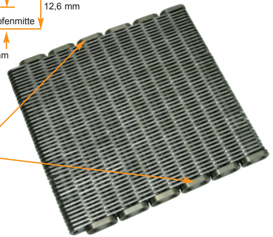
ABB.2) ALLGUARD FX Obere Ansicht
