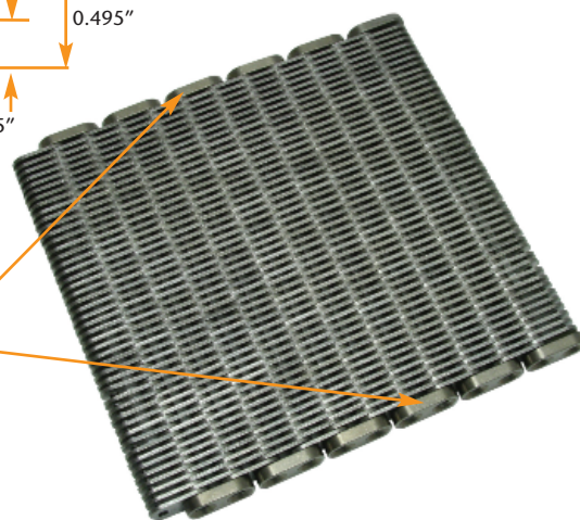
FIGURA 2 ALLGUARD FX Vista de Cima
