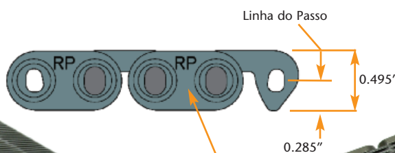
FIGURA 2 ALLGUARD FX Vista de Cima
