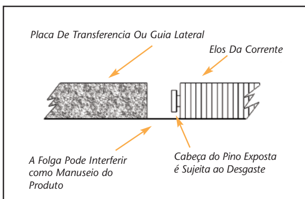
FIGURA 3 Corrente Transportadora Típica
