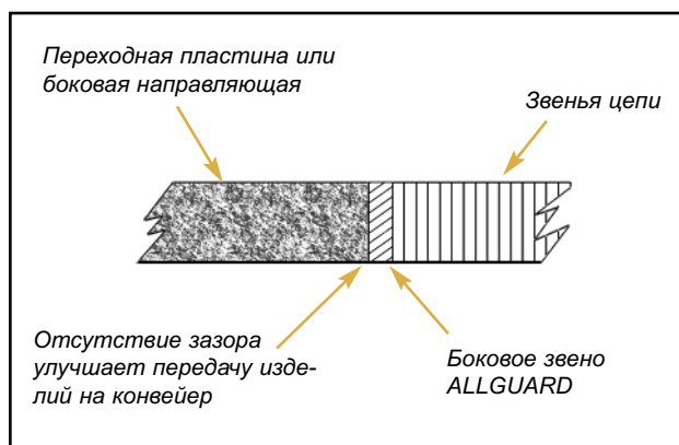
РИС 4 КОНВЕЙЕРНАЯ ЦЕПЬ ALLGUARD
