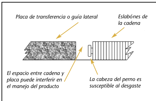
FIGURE 3 CADENA ESTÁNDAR
