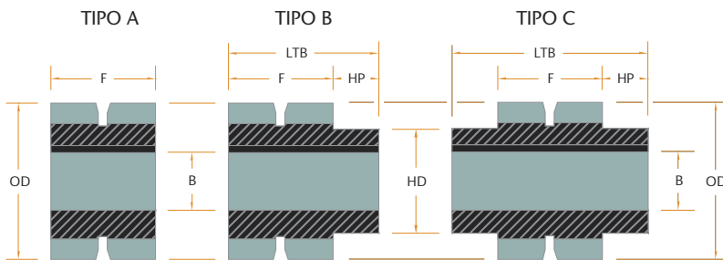
TIPO DE CUBO DEL PIÑÓN
