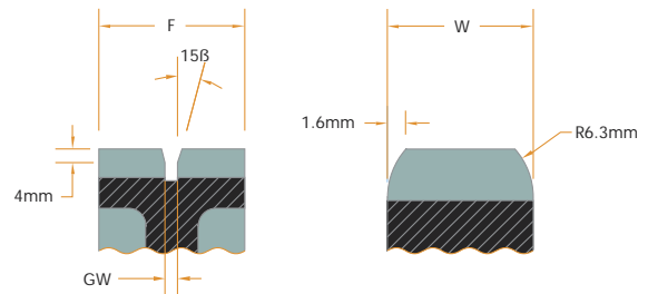
CENTER GUIDE
