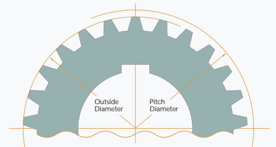
SPROCKET PROFILE
