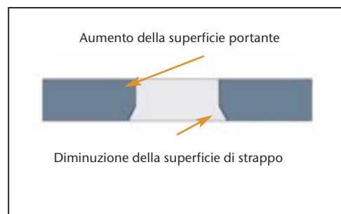
Sezione trasversale dell'apertura di una maglia RP
