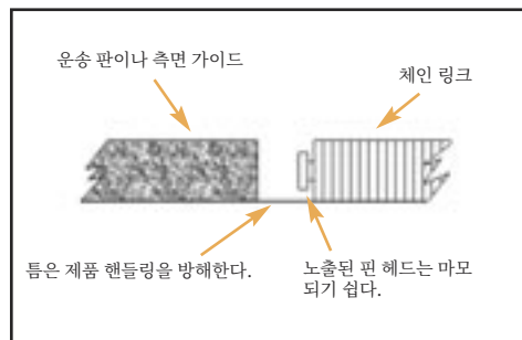
모형1 보통의 컨베이어 체인
