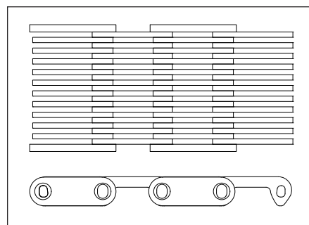
PASSO 1", GUIA LATERAL
