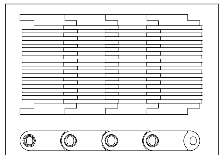
PASSO 1", GUIA LATERAL
