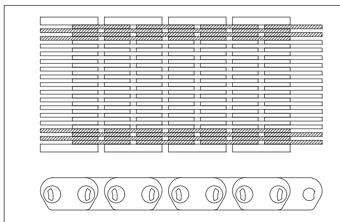
1/2 PULGADA DE PASO, MULTIGUÍA
