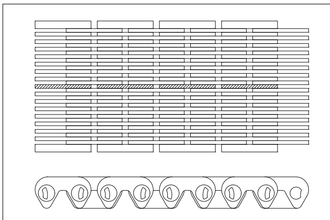
1/2 PULGADA DE PASO, MULTIGUÍA
